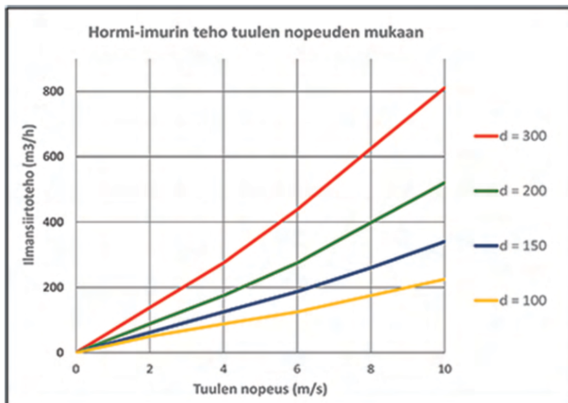
Galvanoitu ja ruostumaton d = 100 mm imuri
