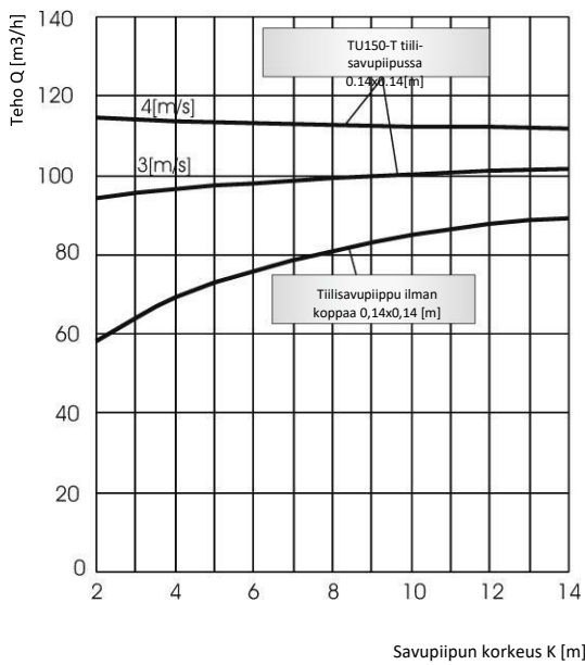
Tehokaavio Turbowent Tulipan Ø150 -malleille savupiipun korkeuden funktiona tiili- tai levymetallisavupiipussa (kaksi tuulen korkeuden funktiona keraamisessa savupiipussa (kaksi tuulen nopeutta: 3 ja 4 [m/s])
