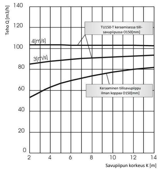
Tehokaavio Turbowent Tulipan Ø150 -malleille savupiipun korkeuden funktiona tiili- tai levymetallisavupiipussa (kaksi tuulen korkeuden funktiona keraamisessa savupiipussa (kaksi tuulen nopeutta: 3 ja 4 [m/s])
